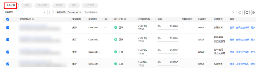
图 4-43 自动扩容
