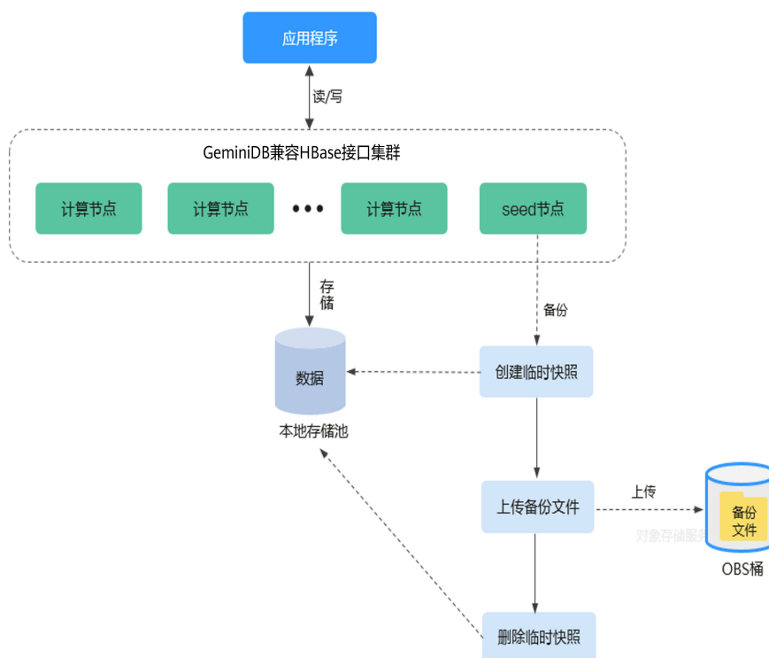
图 4-46 备份原理
