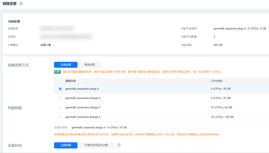
图 4-23 规格变更
