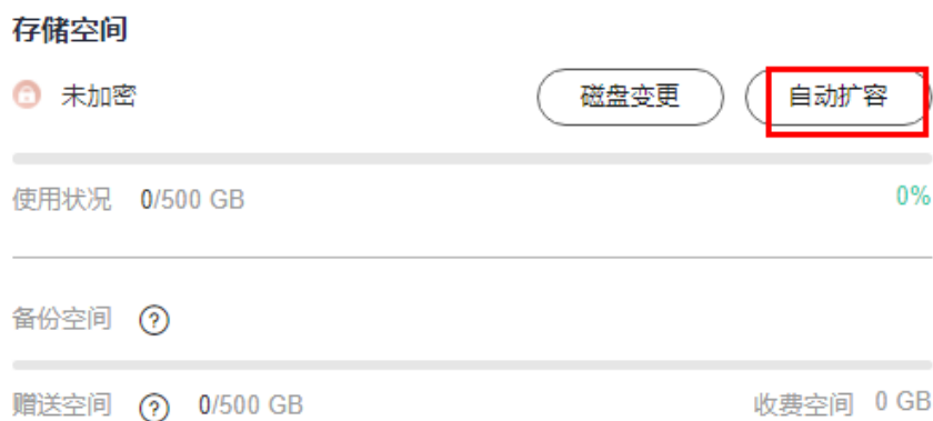
图 4-41 自动扩容
