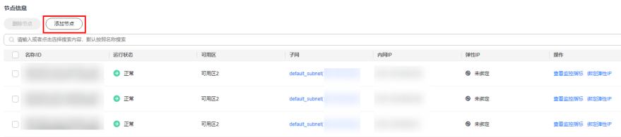
图 4-32 节点信息
